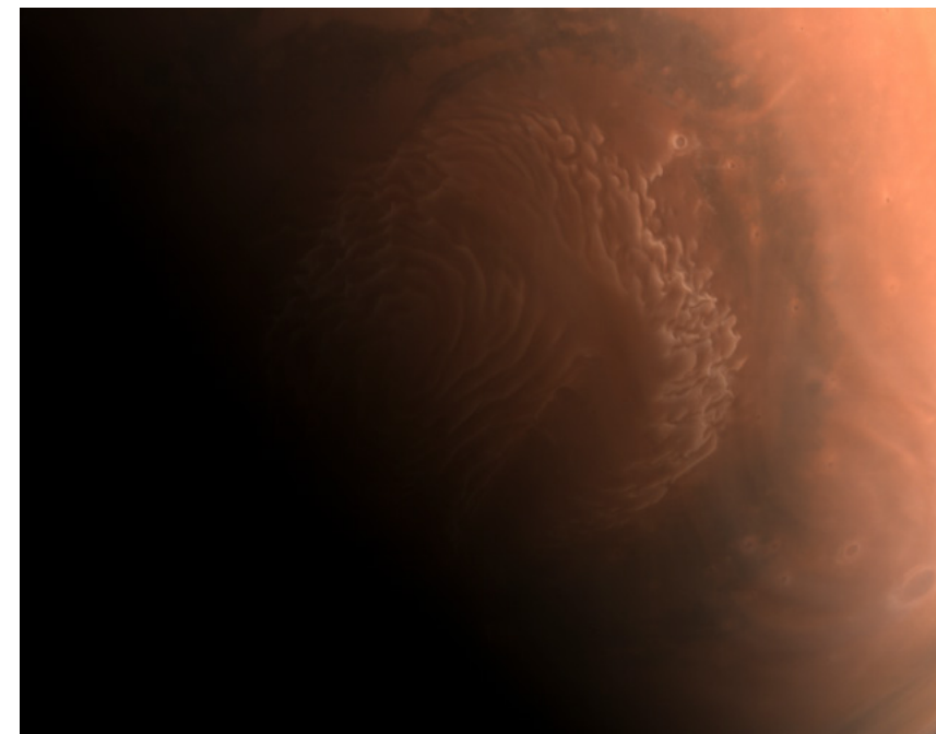
Изображение Марса в высоком разрешении, сделанное китайским зондом «Тяньвэнь-1», 4 марта 2021 г. (фото предоставлено CNSA информагентству Синьхуа)
